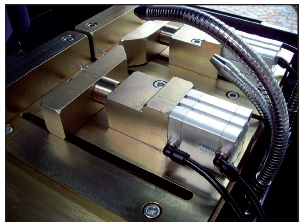
Pneumatischer Spannstock
